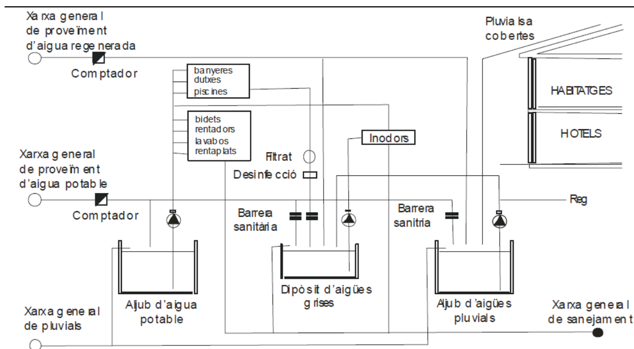
ESQUEMA D'INSTAL·LACIÓ D'AIGÜES GRISSES, REGENERADES I PLUVIALS EN HABITATGES I HOTELS
